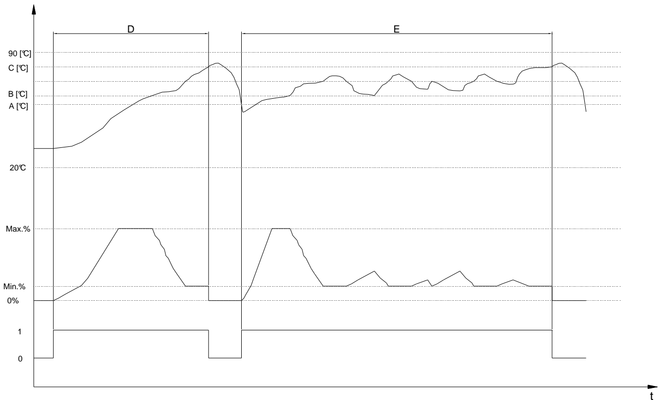
Abbildung – Mögliches Regelverhalten (vereinfachte Darstellung)
