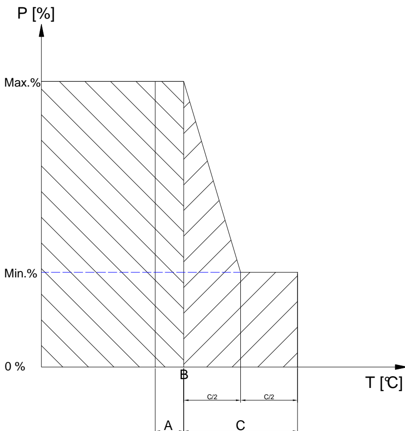
Abbildung – Beispiel für Kesselleistungsregelung (vereinfachte Darstellung)
