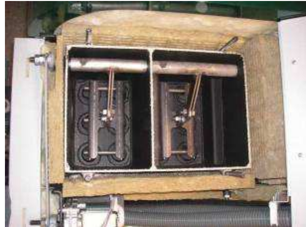
Ansicht auf Wärmetauscherreinigung
