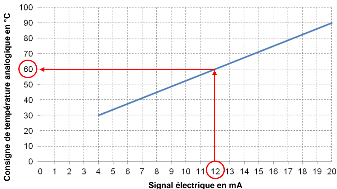
Figure 8.2: Consigne de température analogique en fonction du signal électrique de la demande externe
