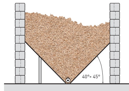
Planchers inclinés glissants avec angle de 40 – 45° dans le silo
