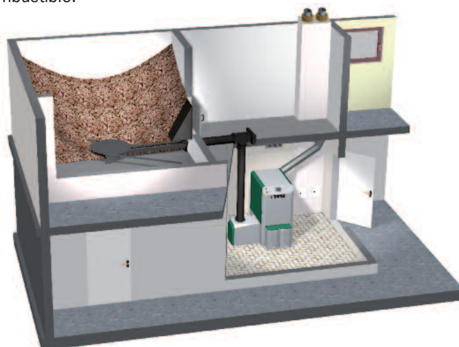
Silo de stockage et chaufferie sur des niveaux différents. Extraction de silo par plateau dessileur rotatif posé à plat et tube de chute par gravité.
