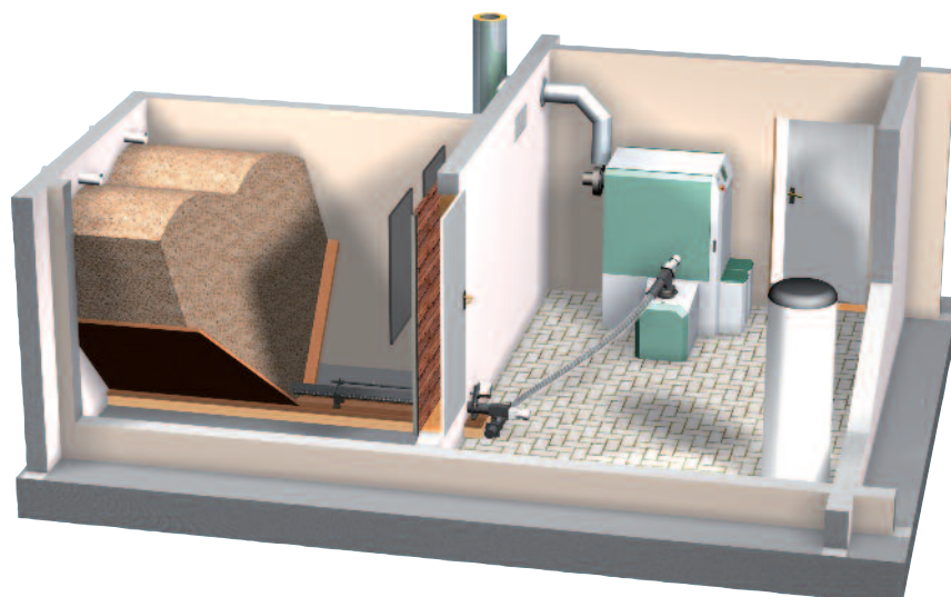
Extraction de silo par vis flexible avec système de reprise
