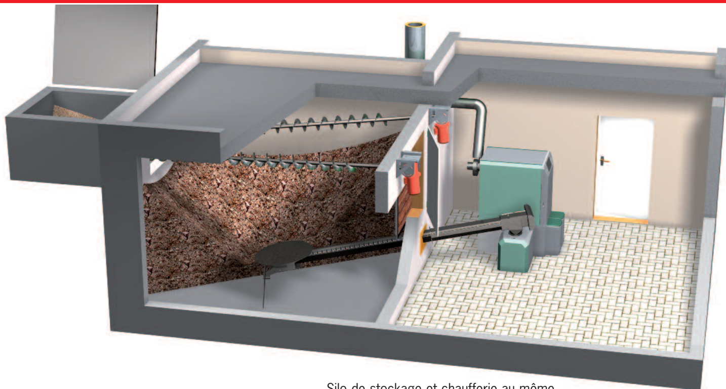
Silo de stockage et chaufferie au même niveau. Extraction de silo par plateau dessileur rotatif posé en pente et 2 vis de remplissage silo.
