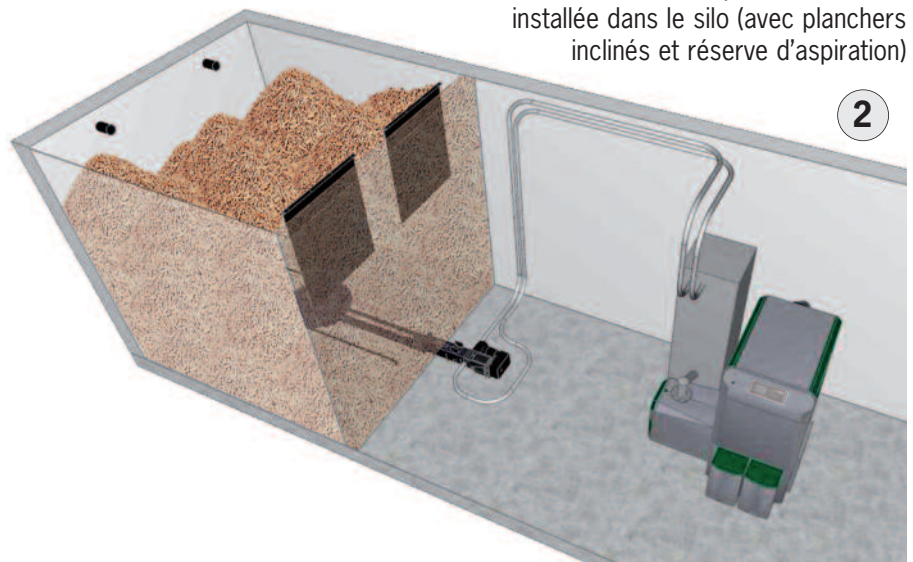
Plateau dessileur rotatif dans le silo avec convoyage pneumatique et réserve d'aspiration. Volume de stockage utile optimisé du fait que les planchers inclinés ne sont pas nécessaires.
