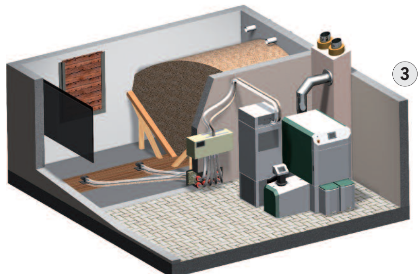
Aspiration multi-points. Le système peut être installé facilement et représente une solution universelle adaptée à chaque configuration de silo.
