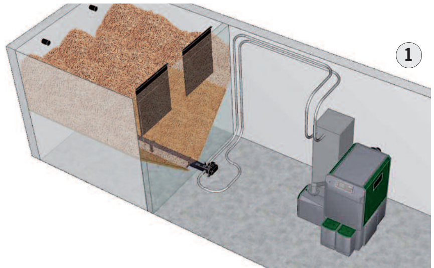
Vis d'extraction pellets modulaire installée dans le silo (avec planchers inclinés et réserve d'aspiration)
