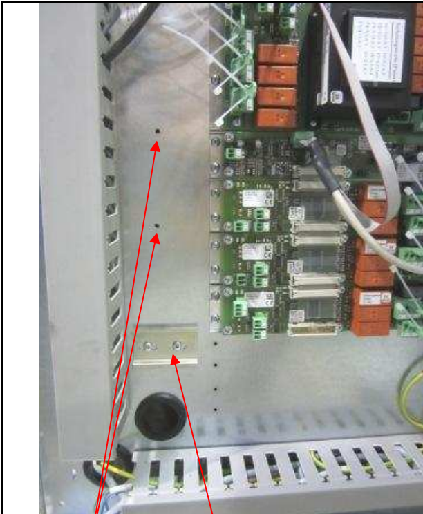
Montage der Schnappschiene für Motorschutz und 2 Bohrungen für Netzfilter. Mount the mounting bar for the engine protection and 2 holes for the mains filter.
