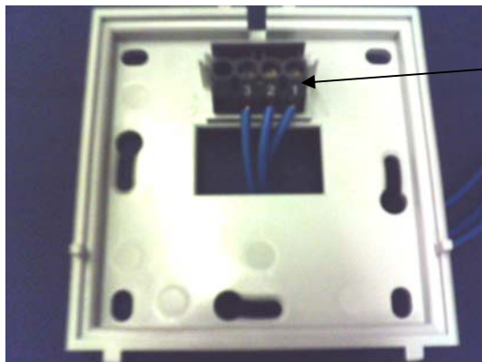
Vue interne de la commande à distance
