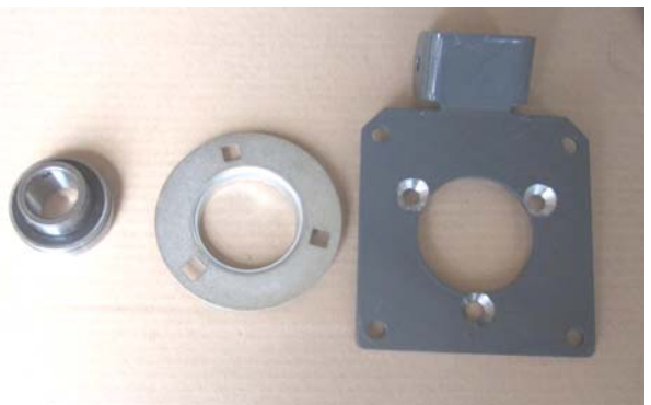
Visser le support de bride avec 3 vis à tête fraisée M8x20, des écrous et des rondelles
