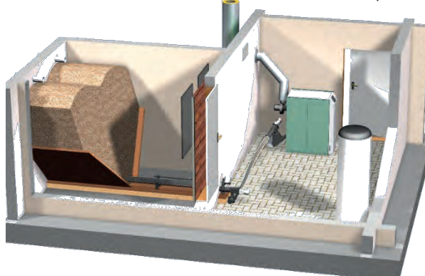
Elément intérieur de silo
