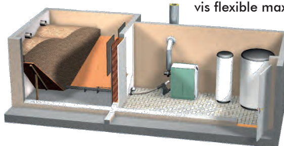
Eléments intérieur de silo
