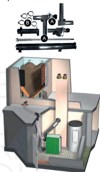
Kit d'extraction pour vis sans fin flexible
