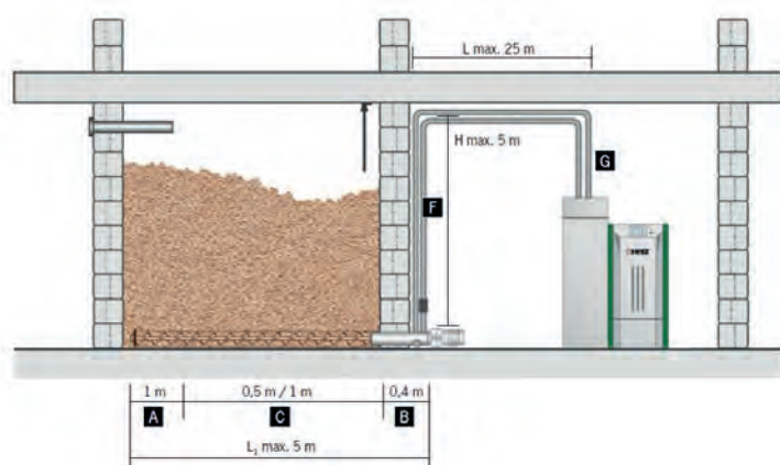
Kit d'extraction pour système d'aspiration par vis sans fin
