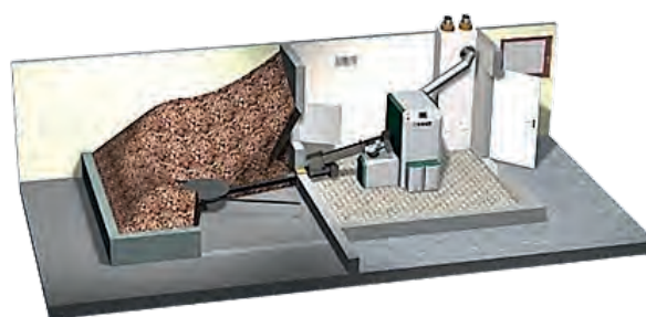
Dessileur avec vis de reprise
