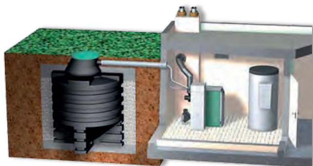
Chaudière Pelletstar avec silo enterré Géotank et transfert pneumatique
